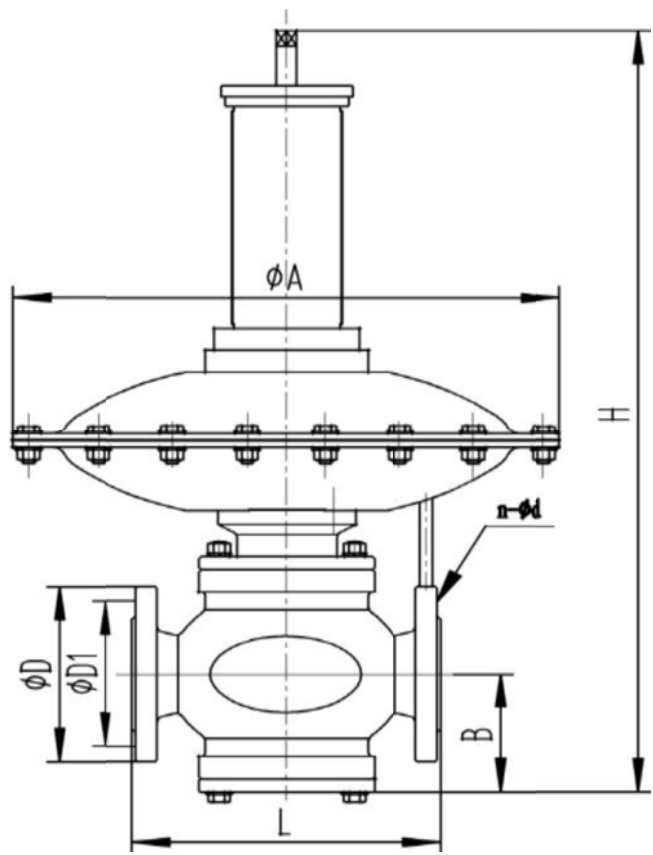
图 2 外形结构
